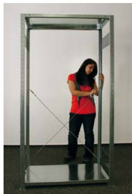
Schritt 4: Diagonale mit Spannschloß einhängen und Regal ausrichten
