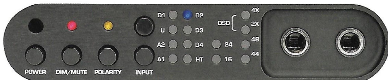
Dicht gedrängtes Anzeigefeld: Über die beiden Inputtasten werden die zwei analogen Eingänge, der USB-Eingang, die vier digitalen Eingänge und der Bypass (HT) geschaltet. Die Wortlänge wird in 16 Bit oder 24 Bit angegeben. Die Samplingrate ergibt sich aus 44 bzw. 48 kHz plus 2 x oder 4 x Oversampling
