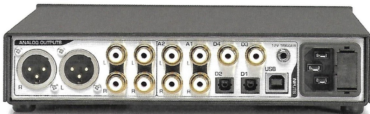
Dicht bepackte Rückseite: ganz links der symmetrische Ausgang sowie die zwei unsymmetrischen Ausgänge. In der Mitte die beiden analogen RCA-Eingänge. Für digitale Quellen stehen zwei optische und zwei koaxiale Eingänge sowie der USB-Eingang zur Verfügung. Rechts der 12 V-Trigger und der Netzanschluss
