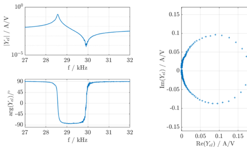
Abbildung 2: Frequenzgangmessung durchgeführt mit dem ATHENA-Generator zur Charakterisierung eines Ultraschallwandlers und der Bestimmung geeigneter Betriebsparameter
