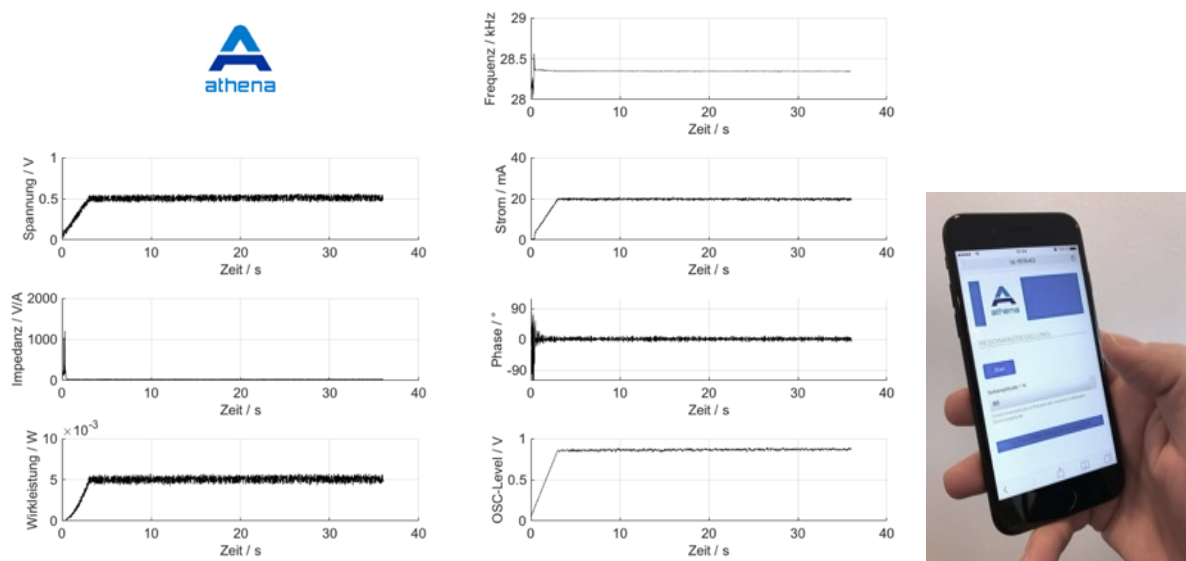
Abbildung 1: Bedieneroberfläche in Matlab zur Prozessüberwachung während des Betriebs eines Ultraschallsystems mit dem ATHENA-Generator (links) und Bedienung des ATHENA-Generators über ein Smart Phone (rechts)
